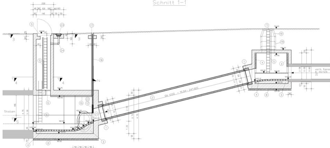
Schnitt 1-1
